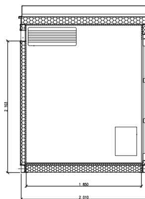
ŘEZ B-B
