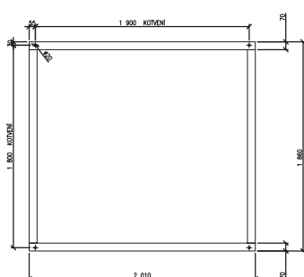
ROZMĚRY RÁMU PRO KOTVENÍ
