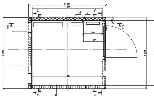
PŮDORYS KONTEJNERU
