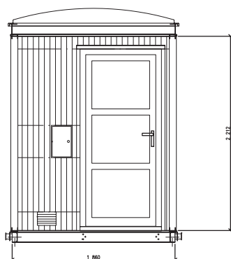
POHLED PŘEDNÍ
